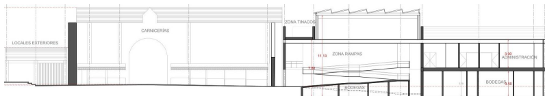
Corte transversal
