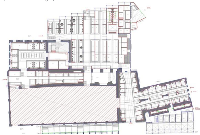
Planta conjunto
