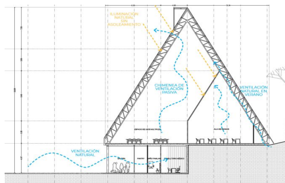
Corte longitudinal
