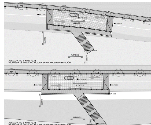
PLANTA TIPO ACCESO AL RÍO
