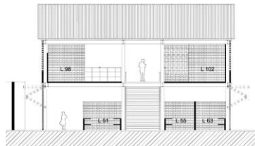
Corte transversal
