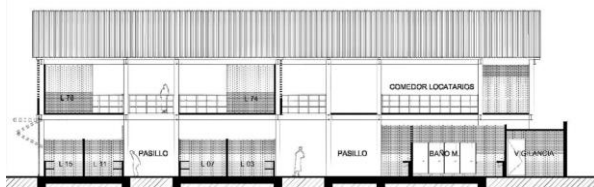
Corte longitudinal
