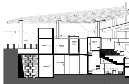
Corte transversal A- A
