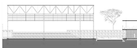
Corte C-C'
