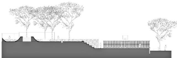
Corte B-B'
