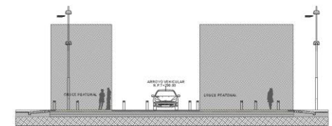
Corte B-B Calle Rascón
