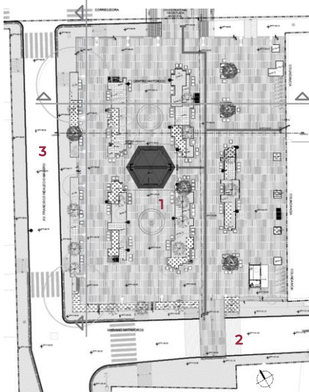
Planta arquitectónica
