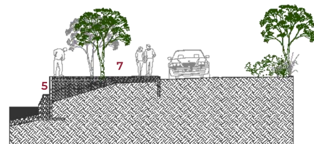
Corte ampliación de banqueta y muro de contención
