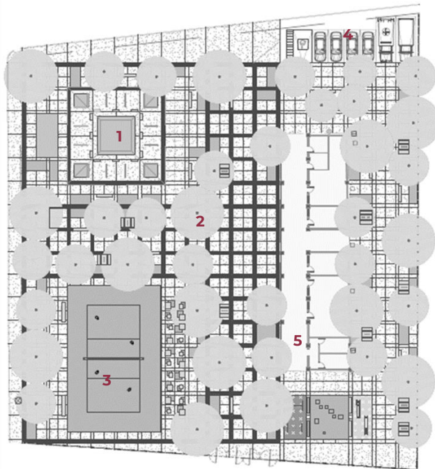
Planta Conjunto
