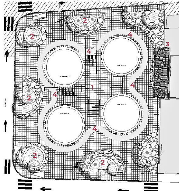
Planta Conjunto
