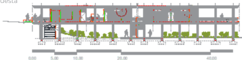
Corte transversal
