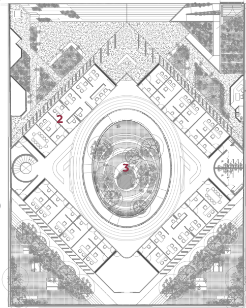
Planta Conjunto
