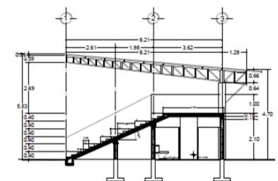
Corte gradas multiusos
