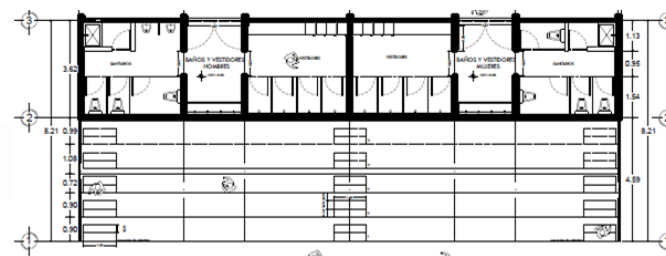
Planta gradas multiusos
