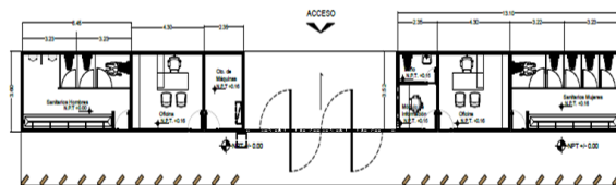
Planta zona administrativa
