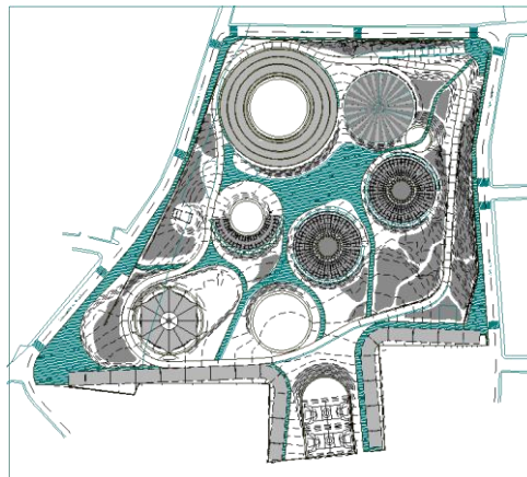
PLANTA GENERAL
