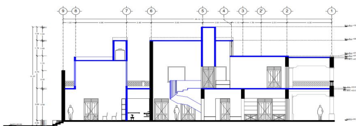
Sección longitudinal
