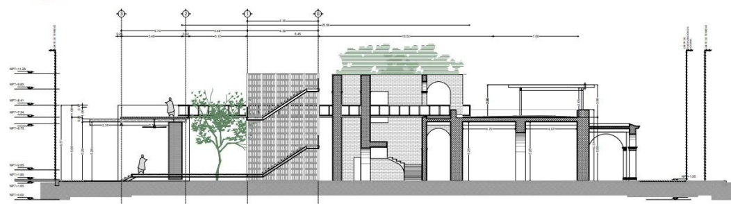
Cortes esquemáticos
