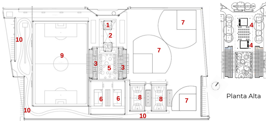
Planta Arquitectónica
