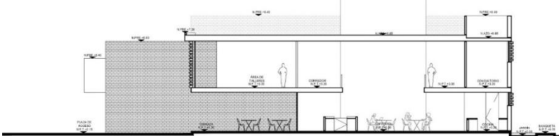
Corte Transversal
