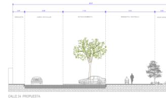
Corte transversal
