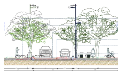
Corte transversal
