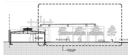
Corte plaza sur
