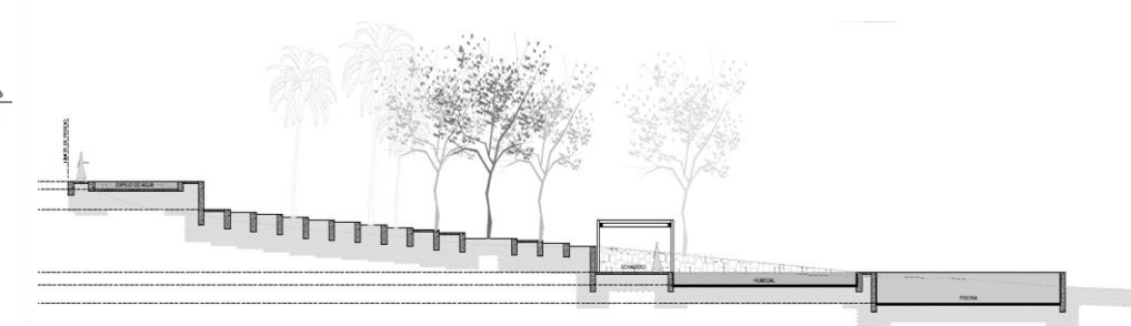
Corte Longitudinal
