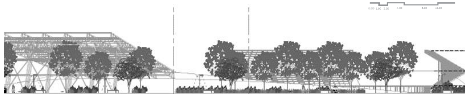
Corte Longitudinal
