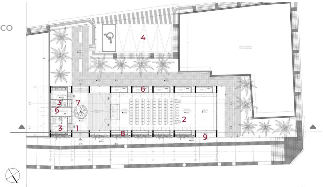
Planta baja
