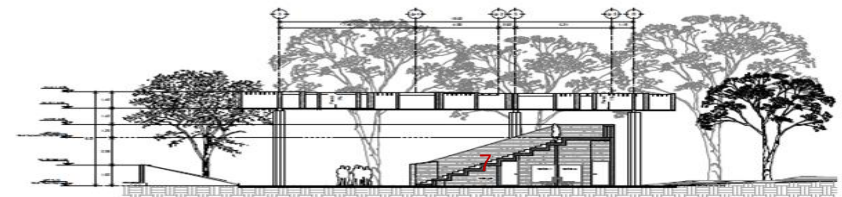
Corte Transversal
