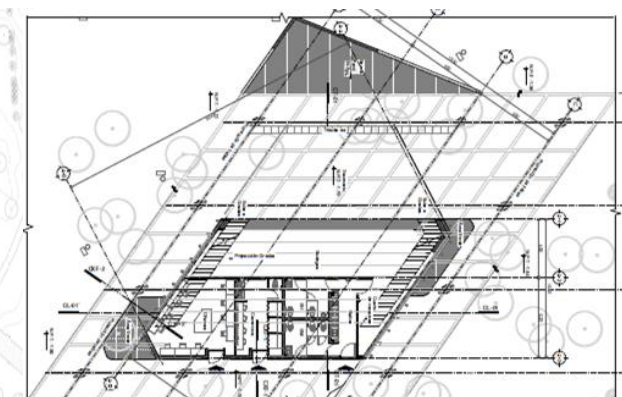
Planta baja
