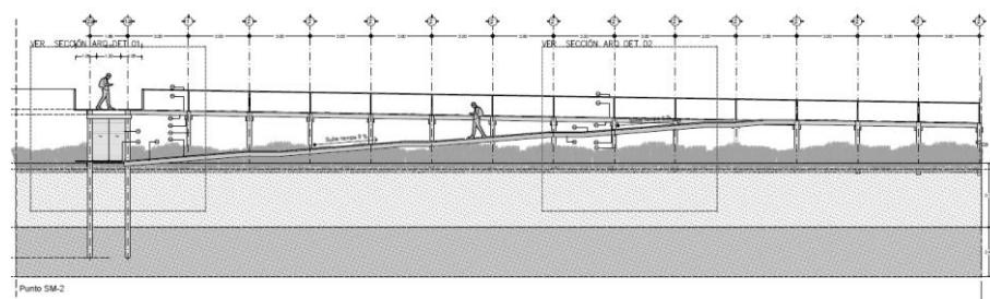
Corte Longitudinal Muelle
