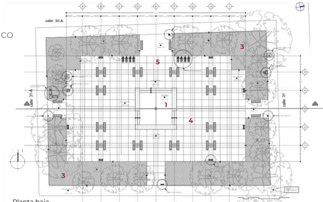
Planta baja
