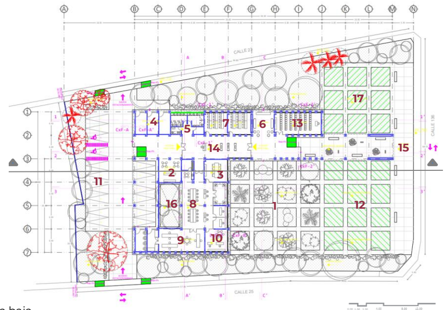
Planta baja
