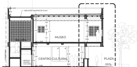
Corte Transversal
