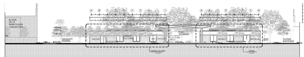
Corte Longitudinal
