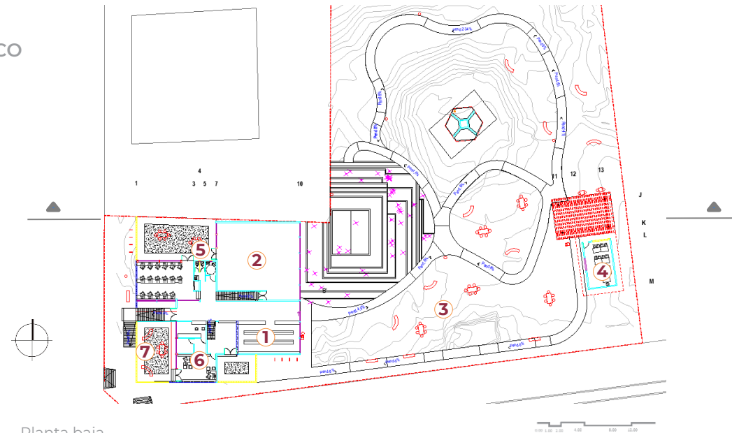
Planta baja
