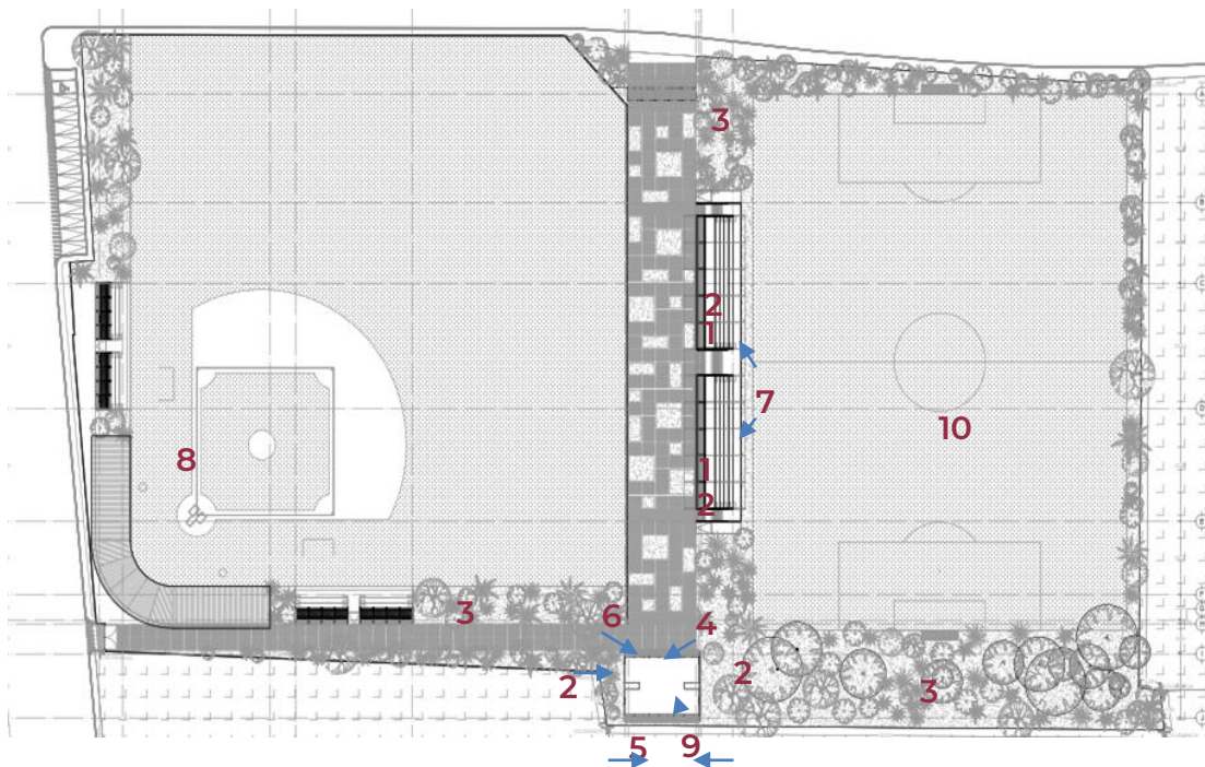
Planta Arquitectónica.
