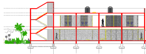
Corte transversal
