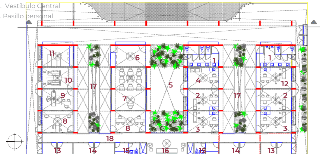
Planta baja
