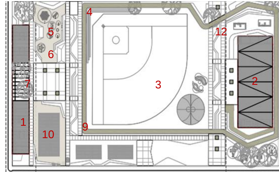
PLANTA ARQUITECTONICA
