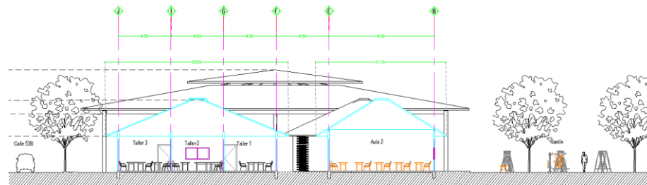
Corte transversal
