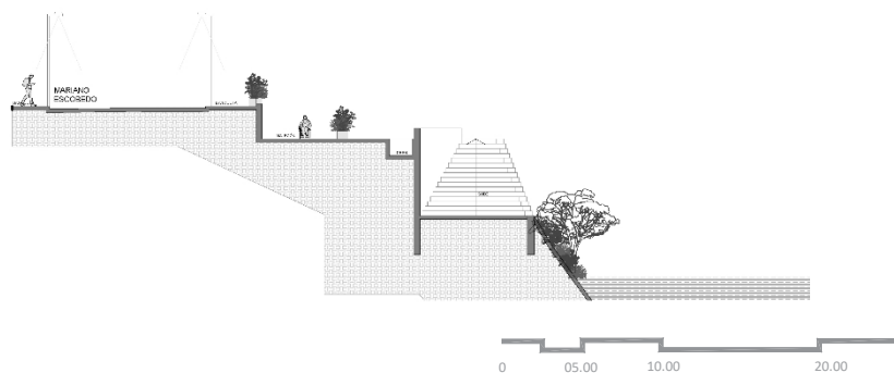
Corte Transversal
