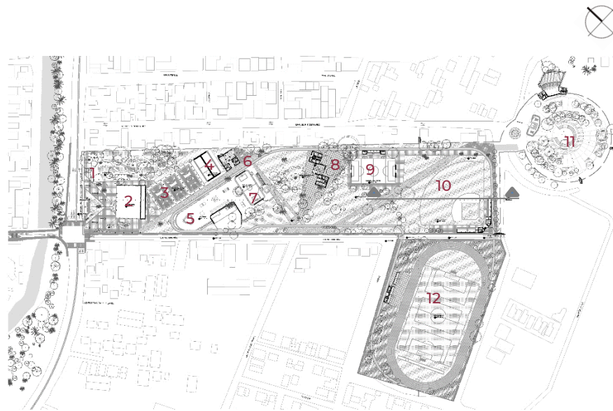
Planta Conjunto
