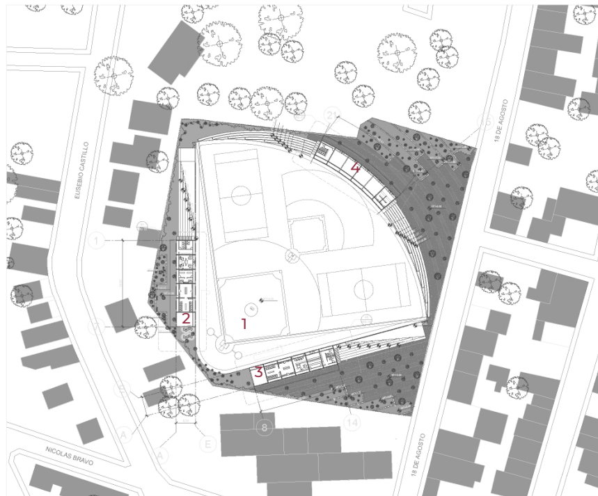
Planta Conjunto
