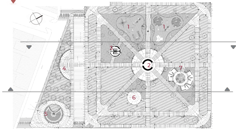
Planta Conjunto
