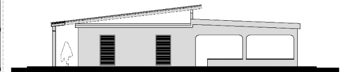
Corte Longitudinal
