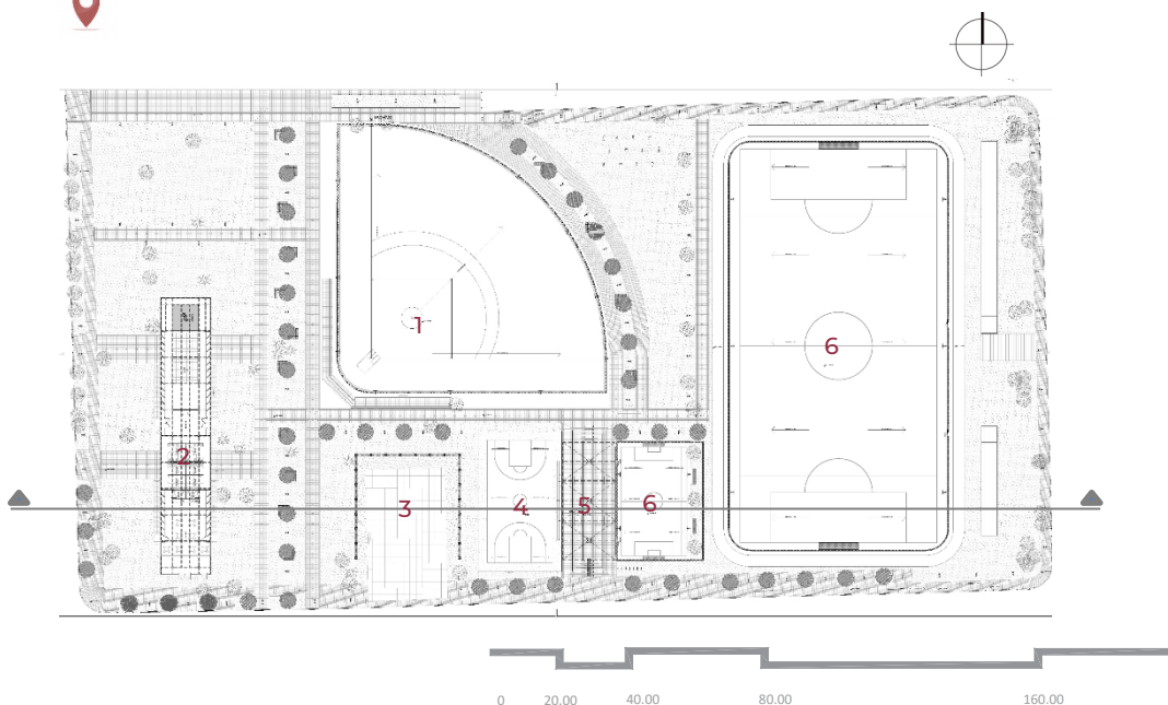
Planta Conjunto
