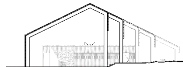
Corte transversal
