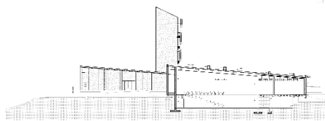
Corte general
