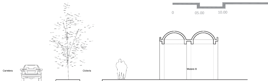
Corte Longitudinal
