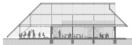
Corte Longitudinal
