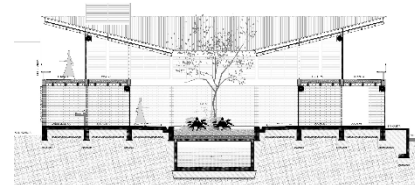
Corte Transversal
