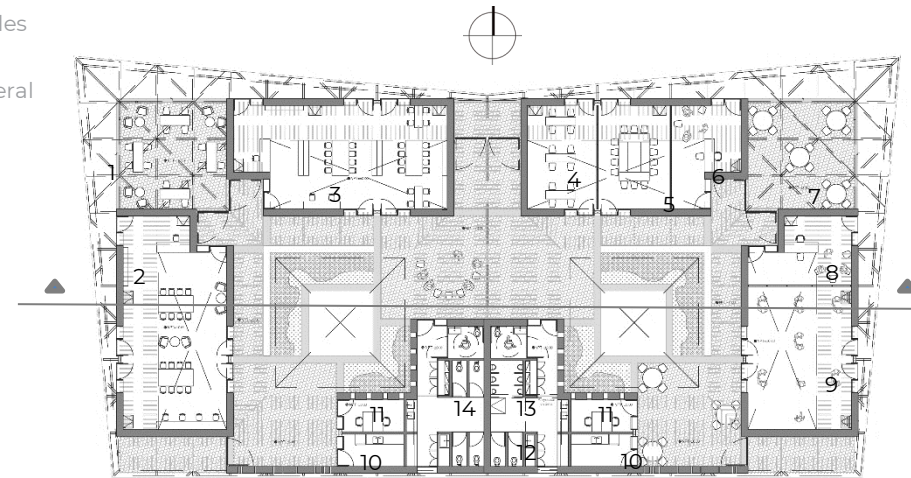
Planta Baja
