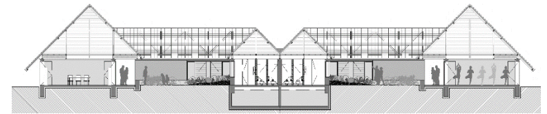
Corte Longitudinal
