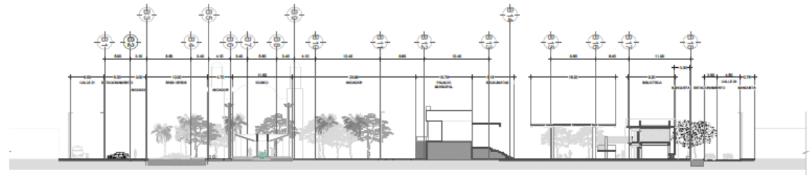
Corte transversal
