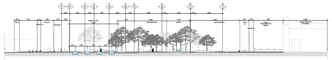
Corte Longitudinal
